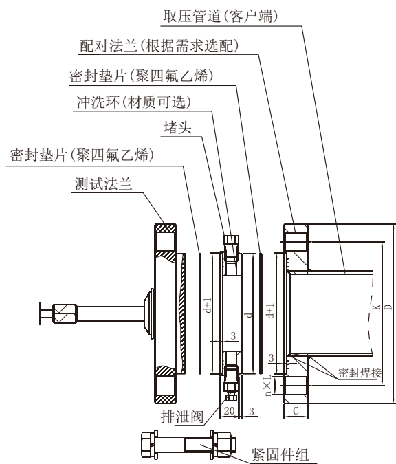
F1/F2 冲洗环
